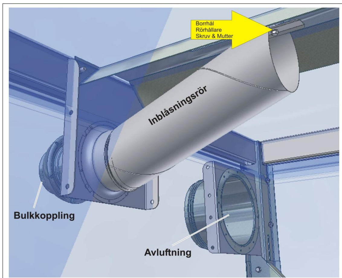
Figur 4: Inblåsningsröret
